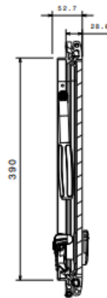
Section A-A Scale: 1:4
