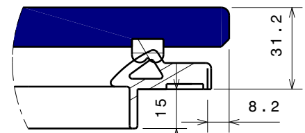
Détail C Echelle : 1:2
