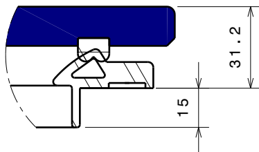
Détail C Echelle : 1:2
